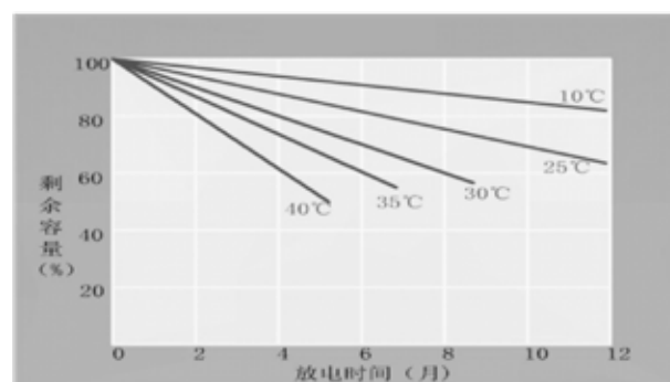
自放电特性
